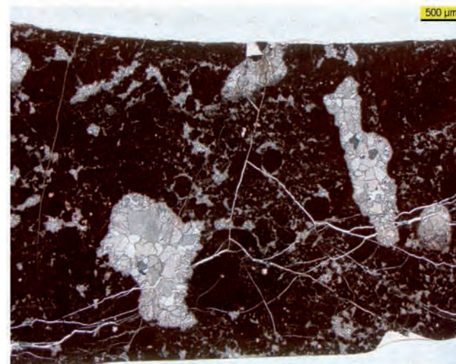
Abb. 6: Lithotyp A, Probe M29, DS//Pol
