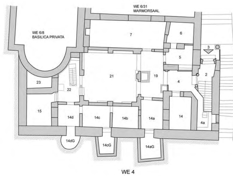
Gegenüberstellung der Grundrisse der WE 1, 2 und 4 in Bauphase IV
