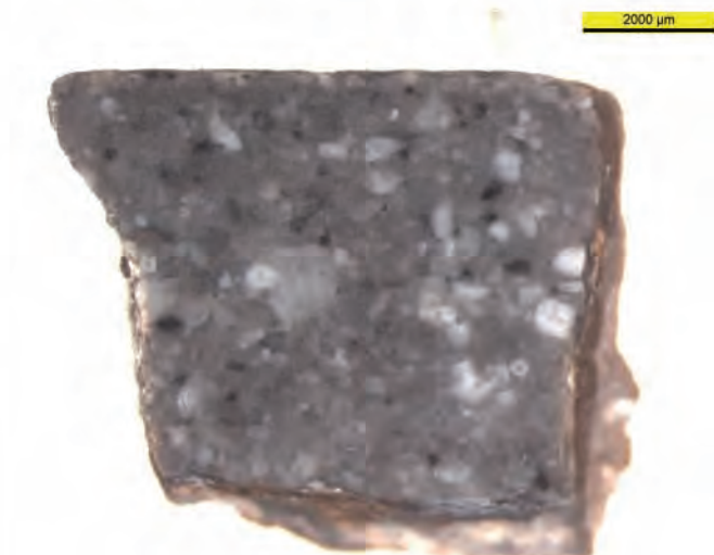
Abb. 40: Lithotyp K, Probe M08c, MF
