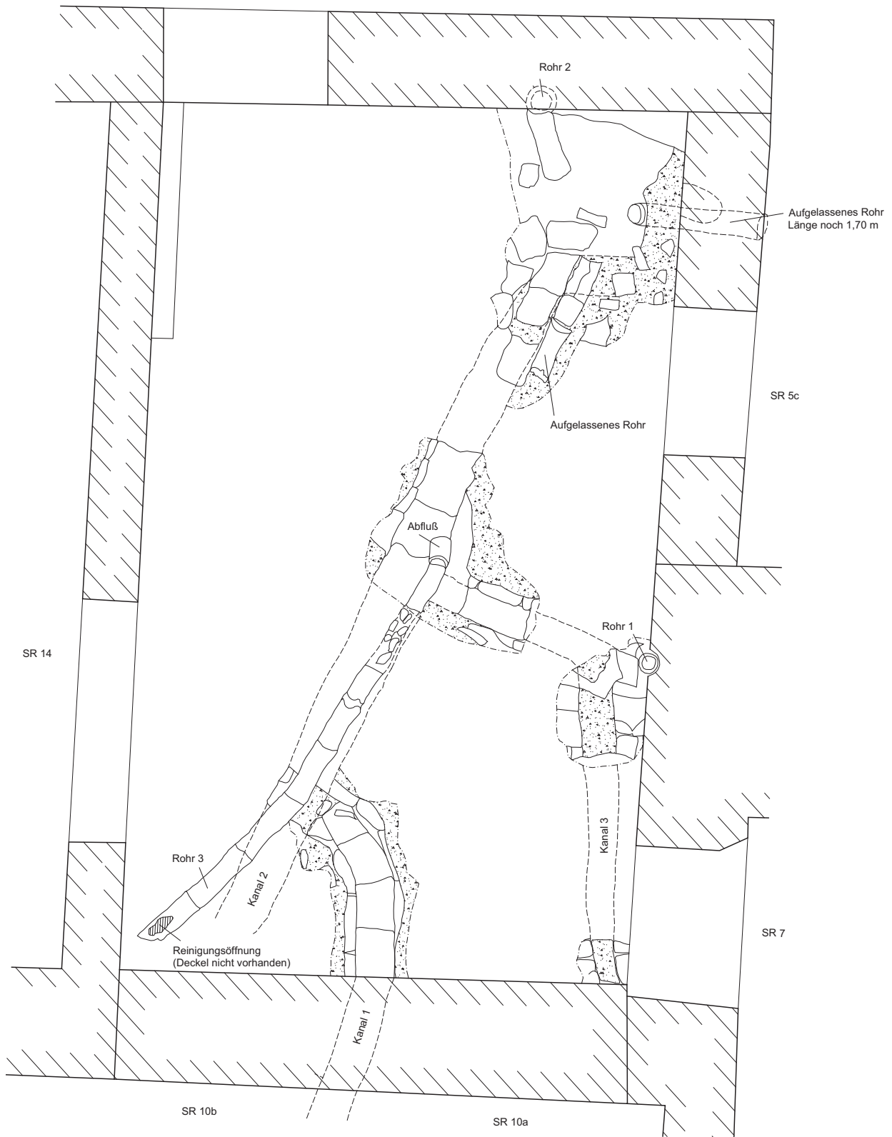
SR 8 Kanalplan Skizze dig.: N.P.
