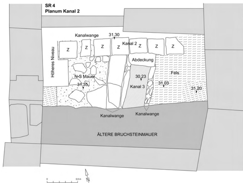
Abb. 43: SR 4, Planum Kanal 2
