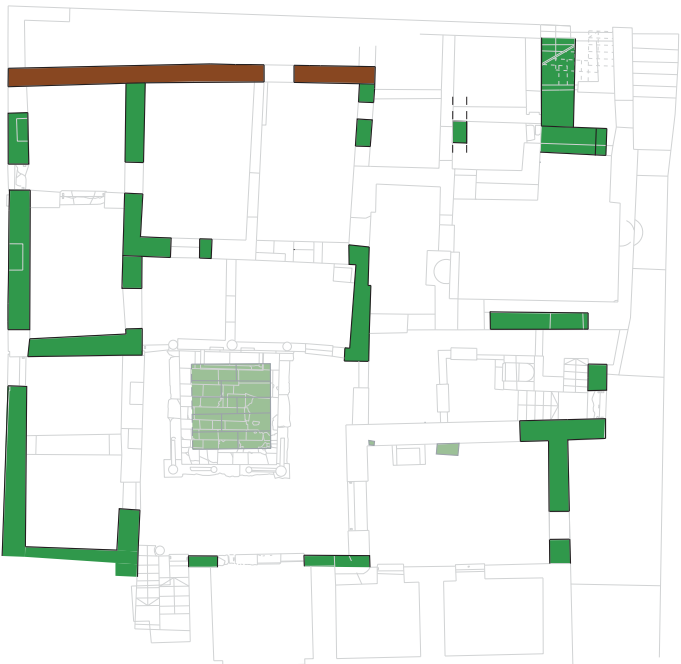
BAUPHASE I - BAUBESTAND
