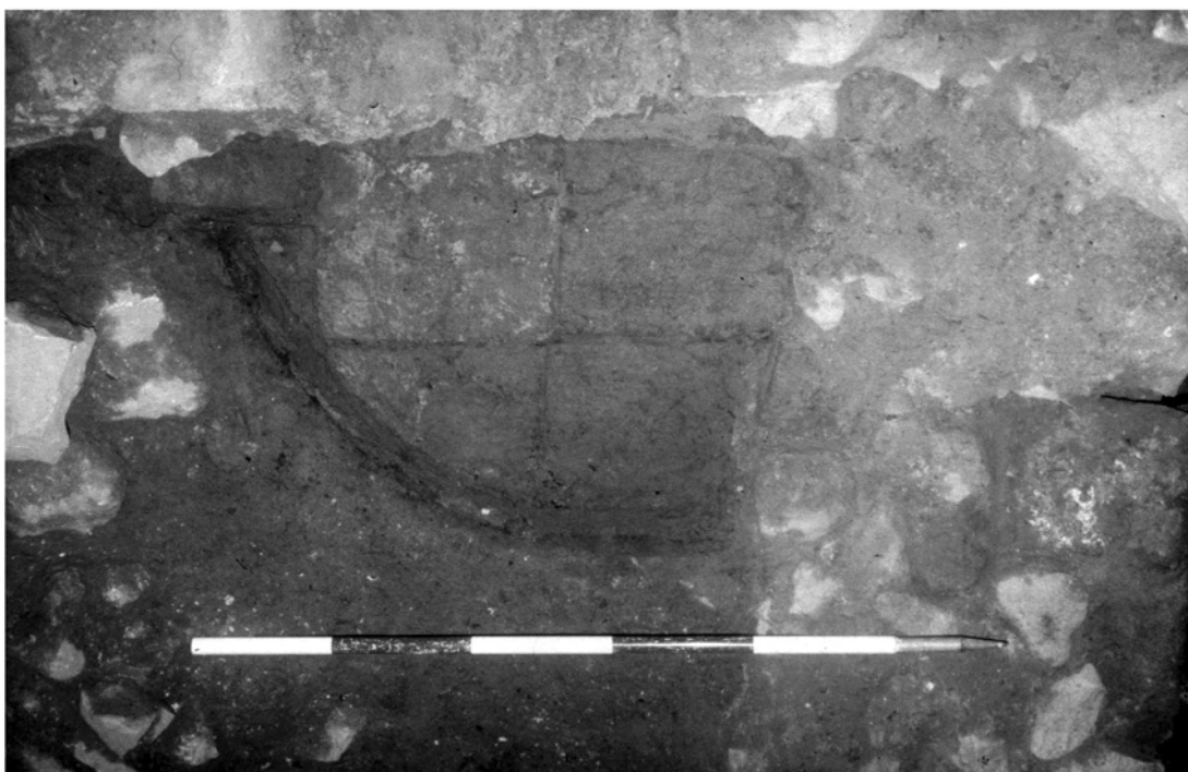
Abb. 6: Ofen 2 – Detail: Bodenplatten und Ofenwand
