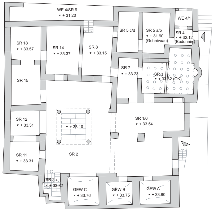
BAUPHASE II - REKONSTRUKTION
