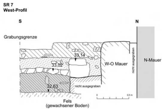
Abb. 10: SR 7 W-Profil mit älterem Gehniveau
