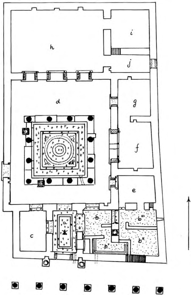
Grundriß des hellenistischen Peristylhauses H 1 und der Maison des dauphin in Delos
