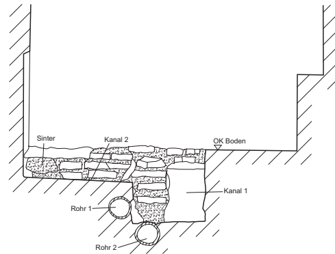
Schnitt A-A
