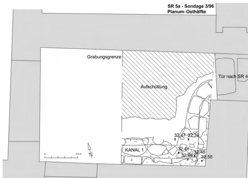
Abb. 56: SR 5a, Sondage 3/96, Planum-Osthälfte
