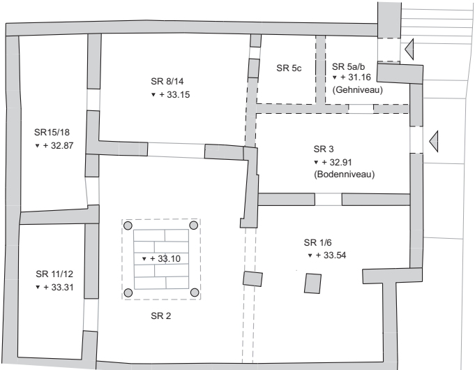
BAUPHASE I - REKONSTRUKTION
