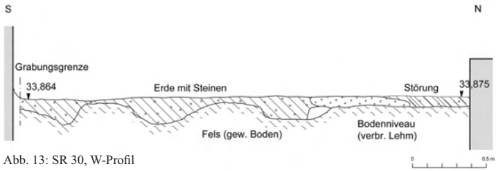
Abb. 13: SR 30, W-Profil
