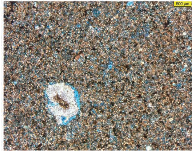
Abb. 44: Lithotyp E, Probe M06a, DS//Pol
