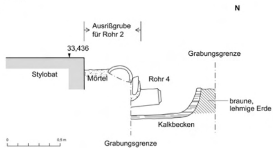
Abb. 15: Schnitt durch Sinterbecken
