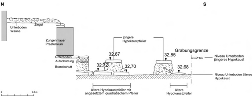
Abb. 29: SR 3, Sondage 1, Schnitt durch Hypokausten
