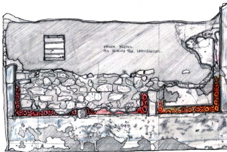
SR 17 NORDWAND
