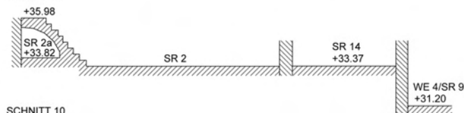
SCHNITT 10
