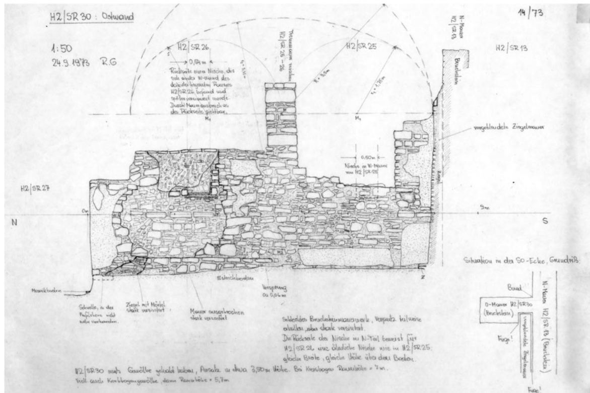
Abb. 4: O-Mauer von SR 30
