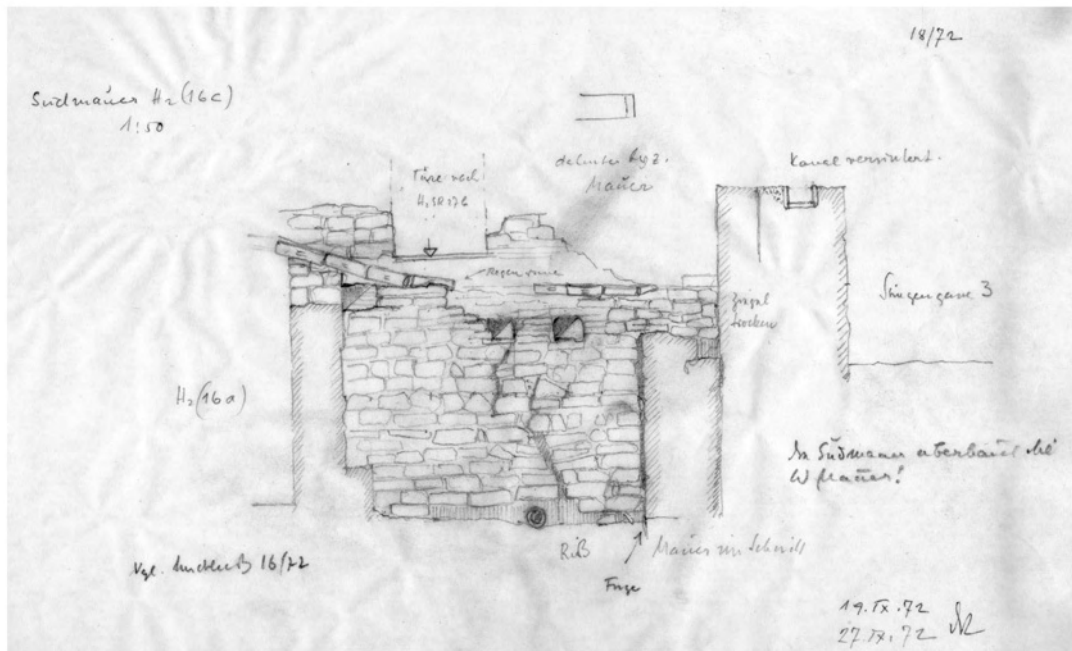
Abb. 16: S-Mauer von 16c mit Tür nach SR 27b
