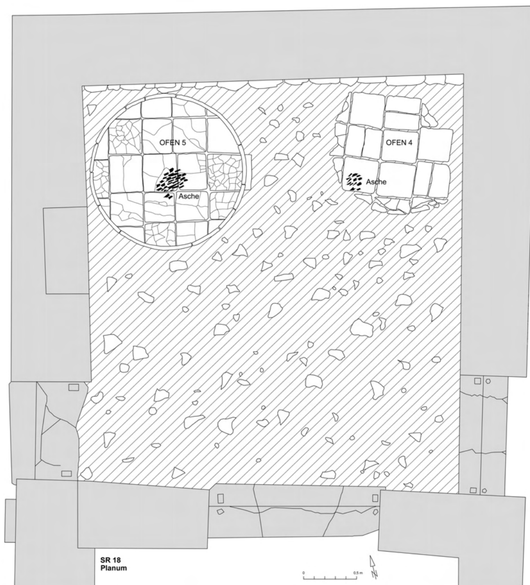
Abb. 20: SR 18, Öfen 4 und 5
