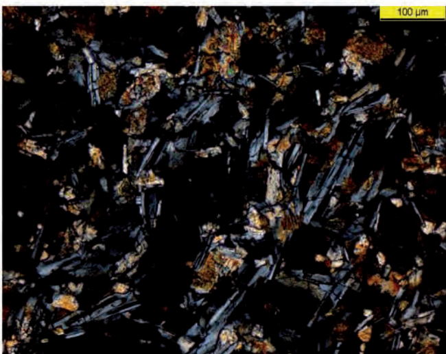
Abb. 21: Lithotyp B, Probe M23b, DS//Pol
