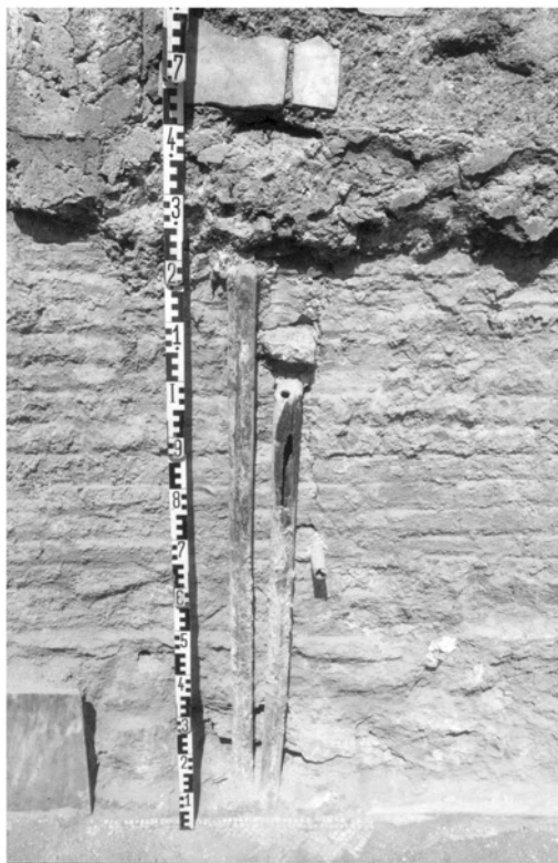
Abb. 11: Bleirohrleitungen des östlichen Brunnens in SR 24 an der N-Wand von SR 22/23
