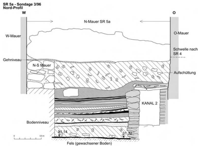
Abb. 58: SR 5a, Sondage 3/96, Nord-Profil
