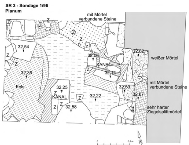
Abb. 12: Sondage 1/96, Befunde der Bauphasen I und II
