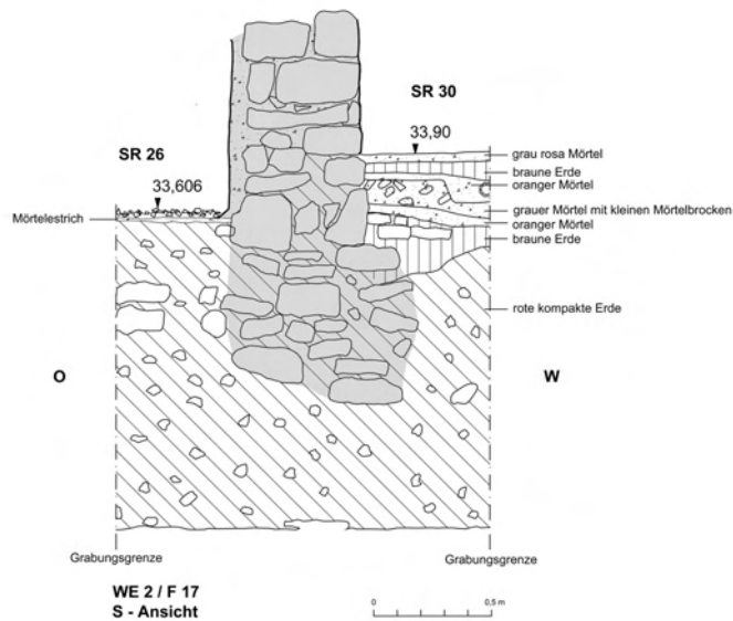
Abb. 27: F 17 – S-Ansicht
