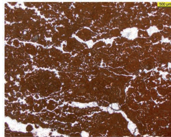
Abb. 4: Lithotyp A, Probe M32a, DS//Pol
