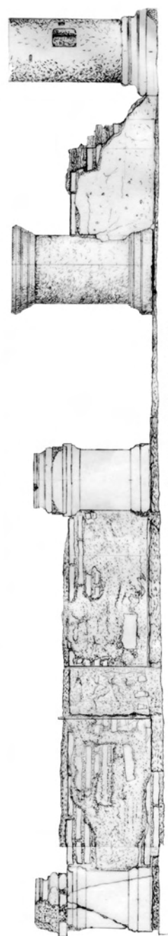
SR 22/23 BRÜSTUNG SÜD (AUSSEN)
