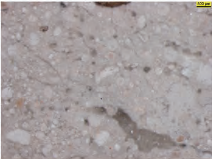
Abb. 10: Lithotyp A1, Probe M20, MF
