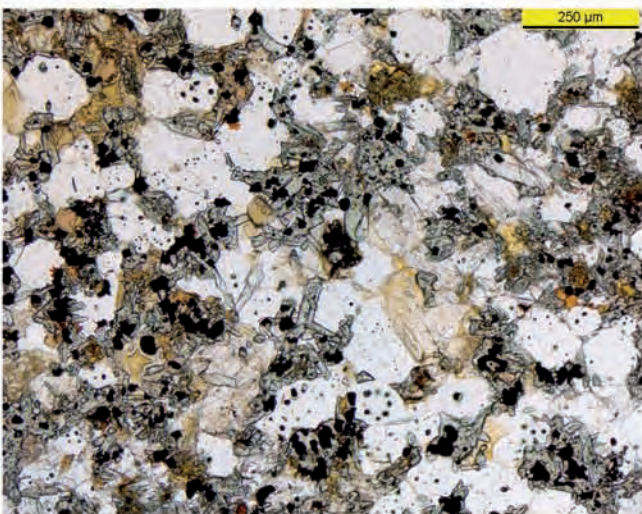
Abb. 23: Lithotyp B1, Probe M09, DS//Pol
