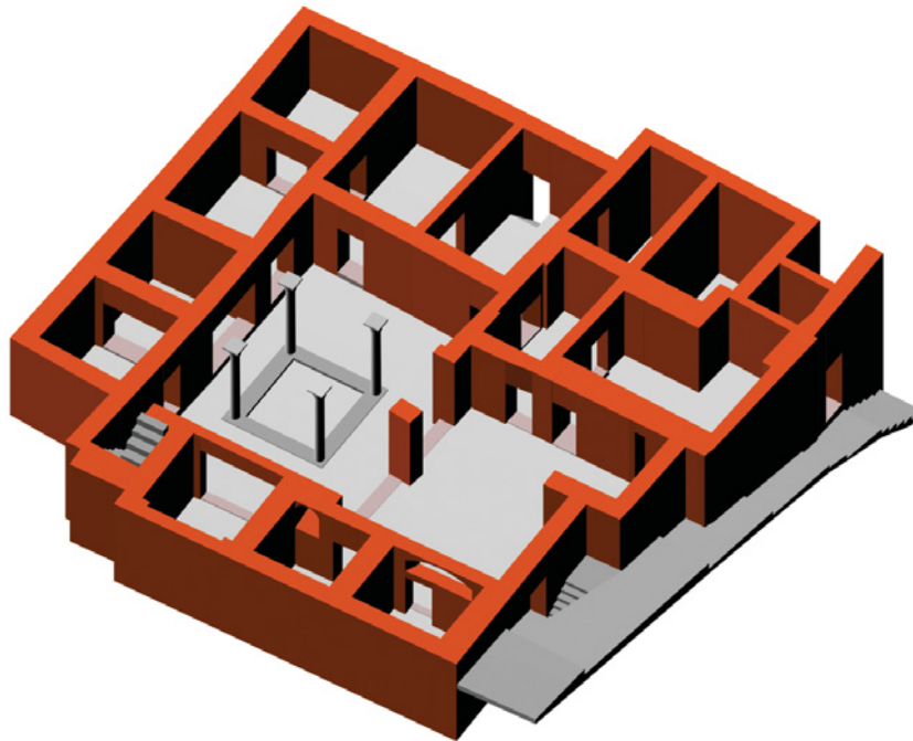
WE 1 ERDGESCHOSS - BAUPHASE II
