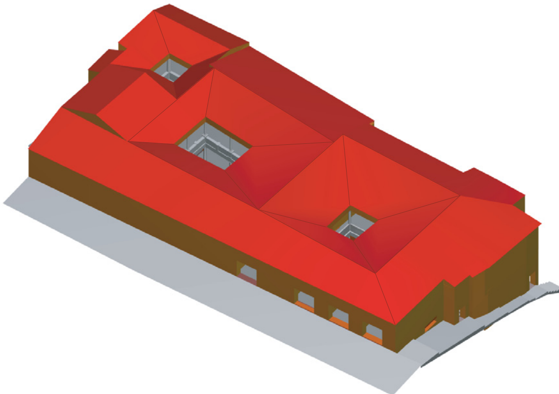
WE 1 & 2 - REKONSTRUKTIONSVORSCHLAG MIT TABERNEN UND DACH
