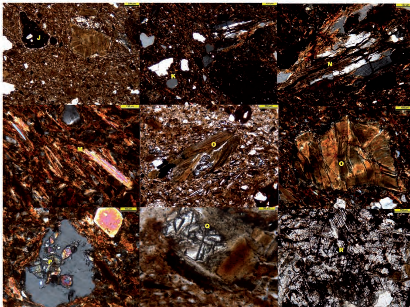
Ofenboden (Typ B) - Dünnschliffübersichtsaufnahme und typische Magerungsbestandteile J: eisenoxidreiche Tonkonkretion; K: Quarzkörner; L: Kristallinbruchstück; M: Detail der glimmerreichen Matrix; N: glimmerreiches Kristallinbruchstück; O: oxidiertes Kristallinbruchstück; P: Feldspat mit Epidot/Klinozoisiteinschlüssen; Q: Klinozoisit führendes Kristallinbruchstück; R: stark verwittertes Marmorbruchstück
