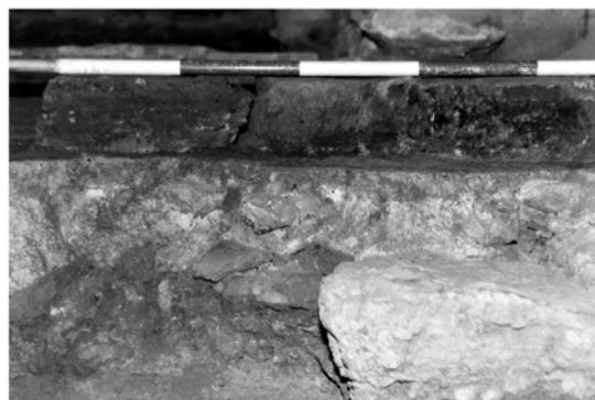
Abb. 23: Unterboden des älteren Hypokausts
