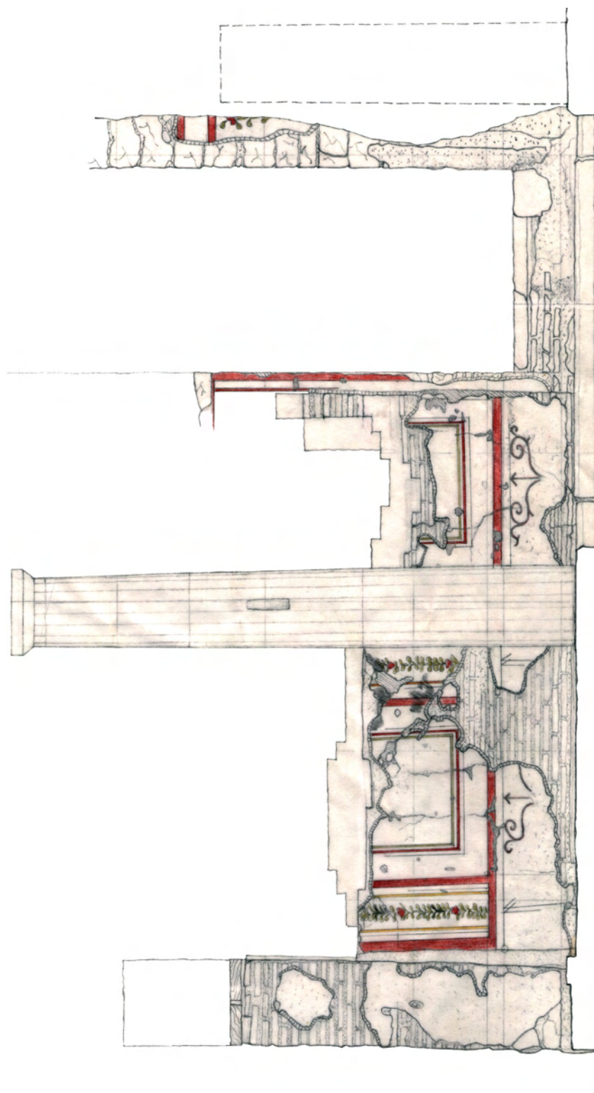
SR 27a NORDWAND AUSSEN
