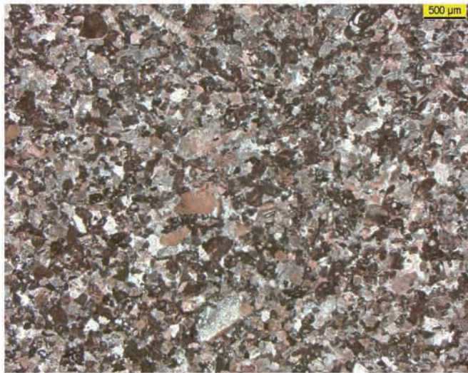
Abb. 14: Lithotyp F, Probe M23a, DS//Pol
