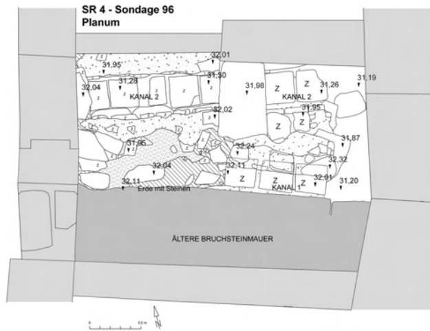
Abb. 41: SR 4, Sondage 96, Planum
