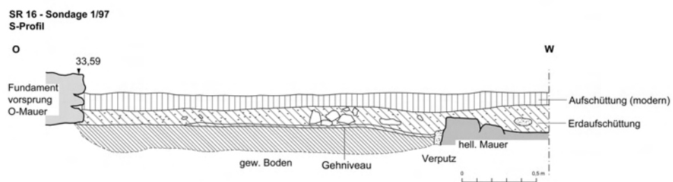
Abb. 2: SR 16, S-Profil
