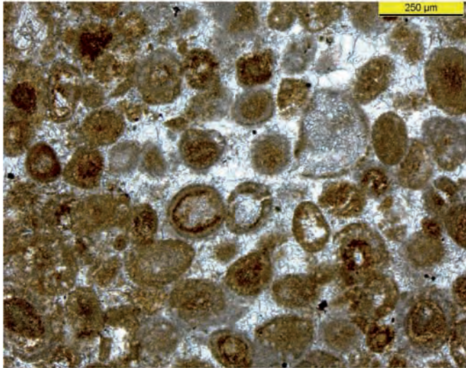
Abb. 42: Lithotyp D, Probe M05, DS//Pol
