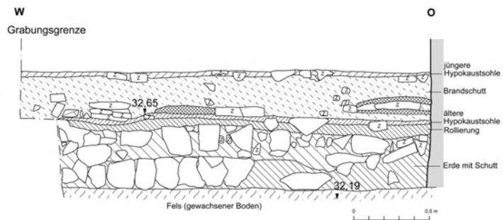
Abb. 13: SR 3, Sondage 1, Nord-Profil
