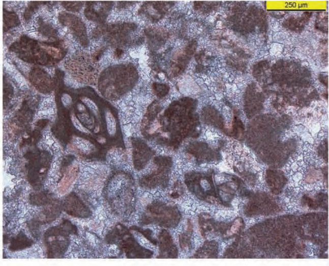
Abb. 16: Lithotyp F1, Probe M17, DS//Pol
