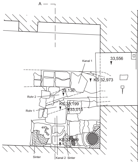
Draufsicht Kanal
