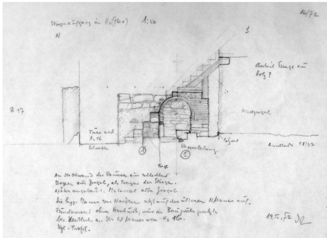
Abb. 15: Stiegenpodest an der O-Mauer von 16c mit rekonstruiertem Verlauf nach SR 27b
