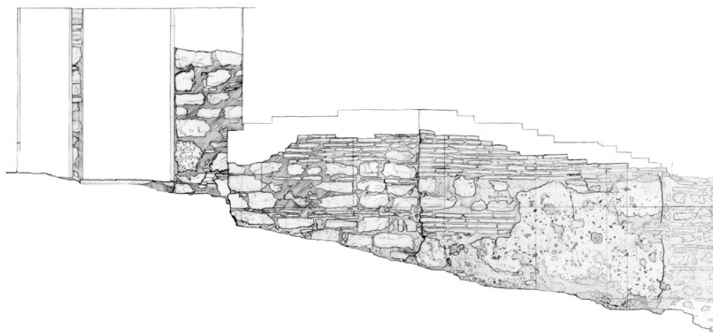
STIEGENGASSE 1 WESTWAND - SÜDL. TEIL
