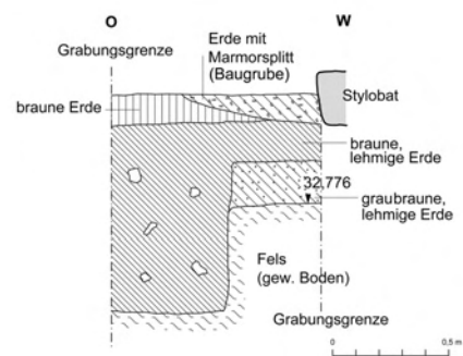
Abb. 10: SR 27, Sondage 5/97, S-Profil
