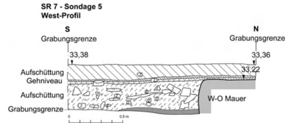
Abb. 72: SR 7, Sondage 5, West-Profil
