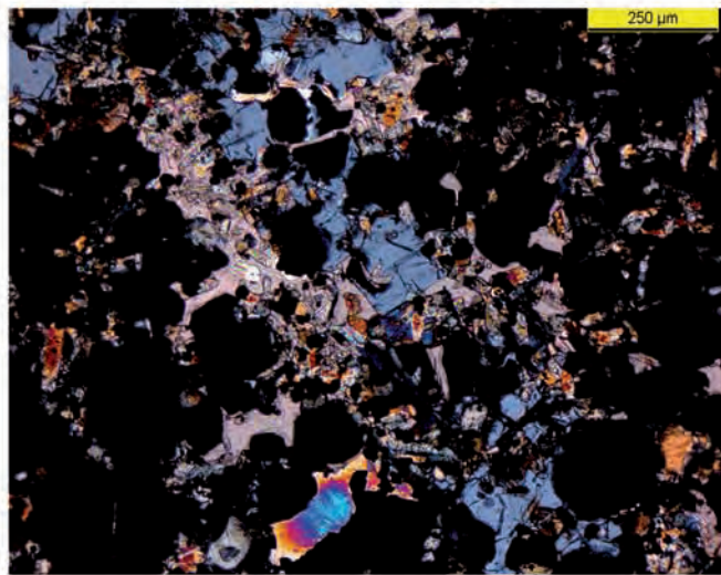
Abb. 29: Lithotyp B1, Probe M28b, DS//Pol
