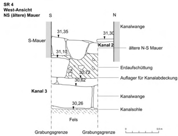
Abb. 47: SR 4 West-Ansicht, NS (ältere) Mauer
