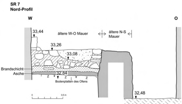
Abb. 71: SR 7, Nord-Profil
