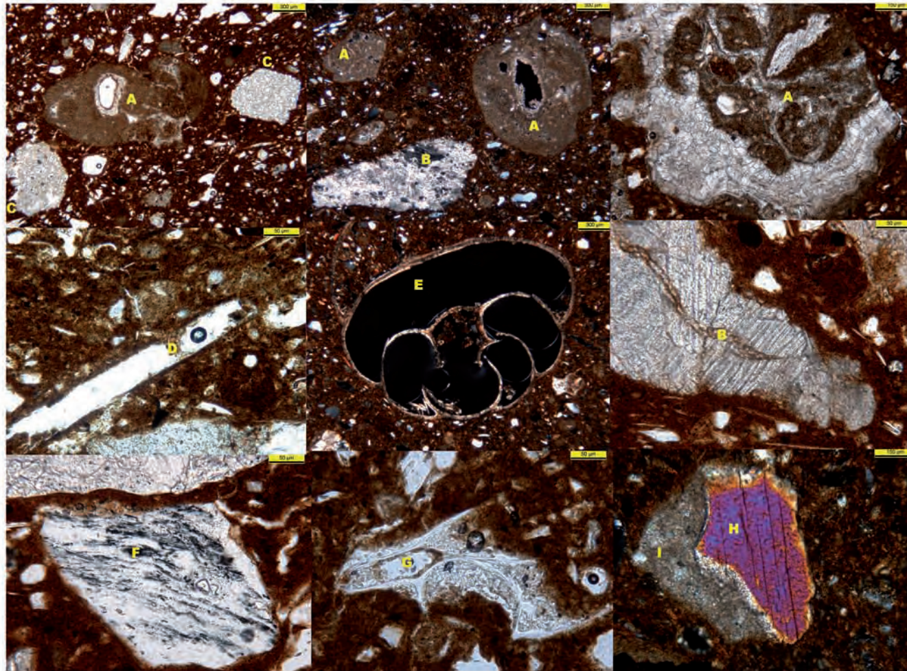
Ofenwand (Typ A) - Dünnschliffübersichtsaufnahme und typische Magerungsbestandteile A: Kalkige Wurzelkonkretion Rizolith; B: Marmorbruchstück; C: sparitischer Kalk; D: Hohlformpore eines ausgebrannten Pflanzenrestes; E: Schneckenquerschnitt; F: typisches Feldspatbruchstück (von Erz durchzogener Albit); G: farbloses vulkanisches Glaspartikel; H: Augitkorn; I: mikritischer Kalk
