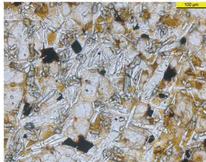
Abb. 20: Lithotyp B, Probe M23b, DS//Pol
