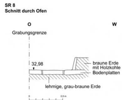
Abb. 19: Schnitt durch Ofen 3
