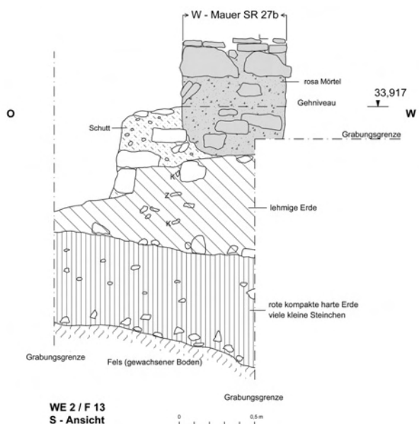
Abb. 25: F 13 – S-Ansicht
