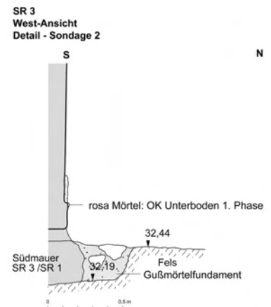
Abb. 7: SR 3, West-Ansicht, Detail – Sondage 2
