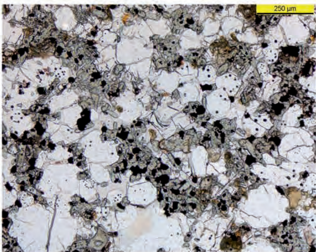
Abb. 28: Lithotyp B1, Probe M28b, DS//Pol
