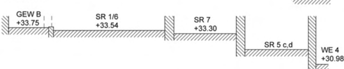
SCHNITT 11
