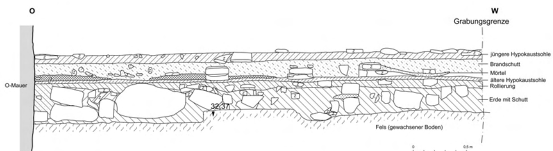
Abb. 28: SR 3, Ostprofil
