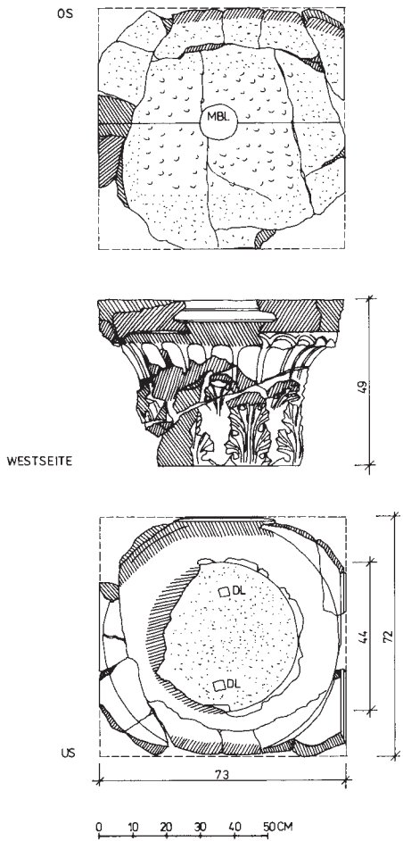
Abb. 18: Kapitell A32
