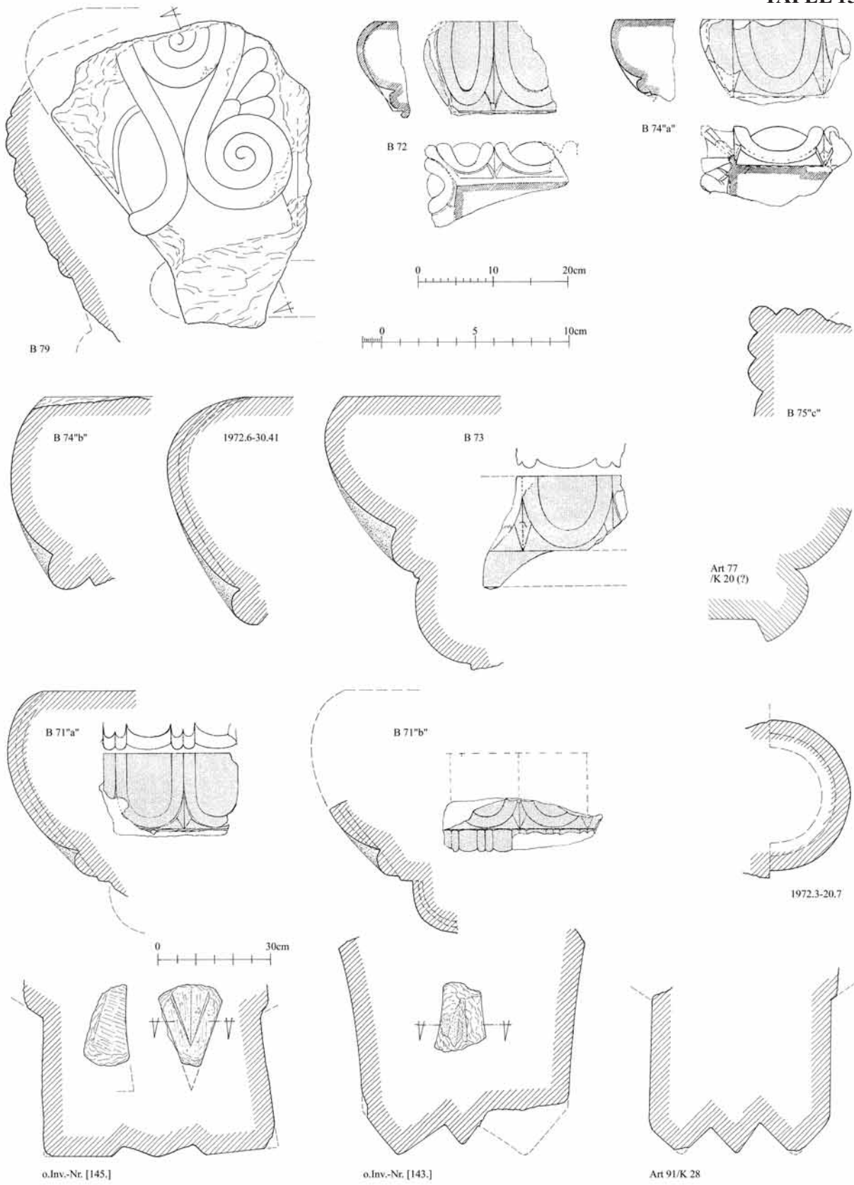
Fragmente von ionischen Kymatien vom Abakus (z.T. nach A. E. Henderson) sowie ein gekrümmtes Perlstabfragment – Kat. 211–216, 219, 234, 259–261, 269 und 2 ohne Kat.-Nr. (B 71 „a, b“, 72, 73, 74 „a, b“, 75 „c“, 79; 1972.3-20.7, 1972.6-30.41; ohne Inv.-Nr. [143.], [145.]; Art 77/K 20(?), 91/K 28) – M. 1 : 2, 1 : 5 und 1 : 10
