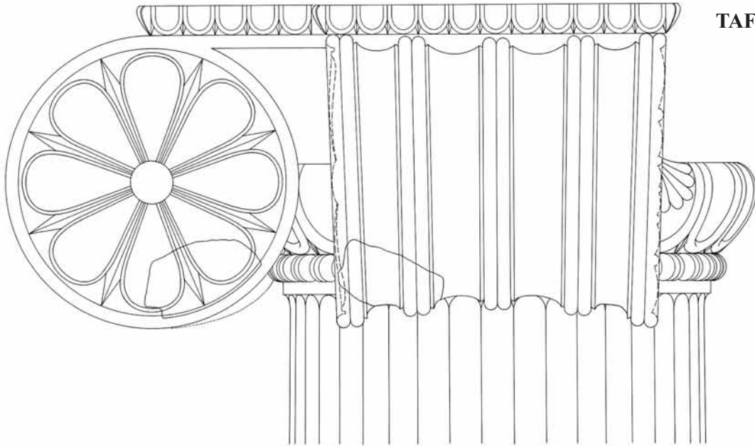
Rekonstruktionszeichnung eines an der Innenecke mit Rosetten geschmückten Kapitells (neues Fragment in der Seitenansicht zweimal eingezeichnet) – M. 1 : 12,5
