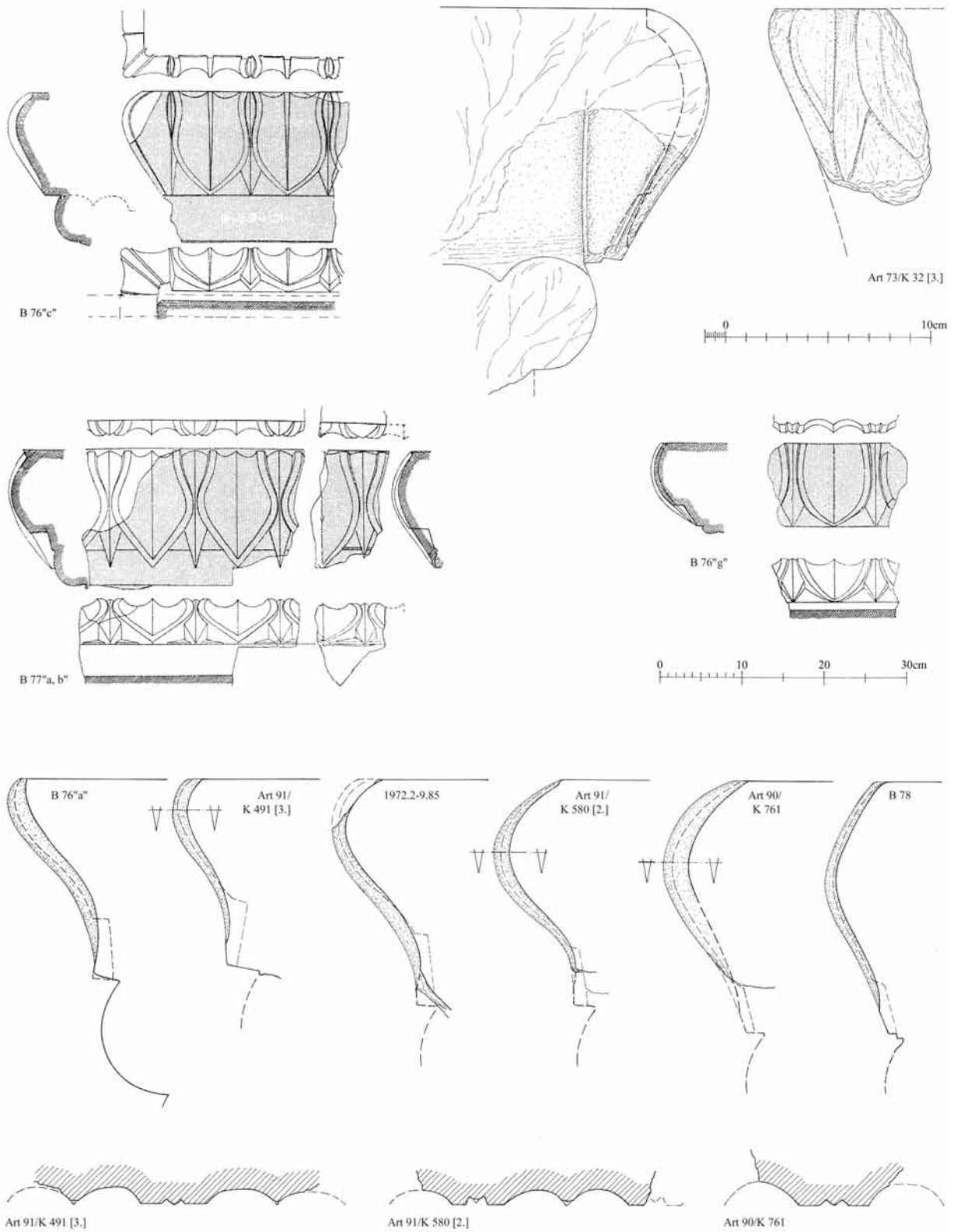
Fragmente von lesbischen Kymationen vom Abakus (z.T. nach A. E. Henderson) – Kat. 223, 225, 229–231, 233, 237–240 und 1 ohne Kat.-Nr. (B 76 „a. c“ und „g“, 77 „a. b“, 78; 1972.2-9.85; Art 73/K 32[3.], 90/K 761, 91/K 491[3.], 91/K 580[2.]) – M. 1 : 2 und 1 : 5
