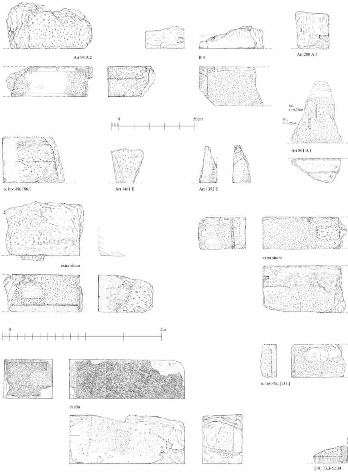
Vollständiger und fragmentarische Quader – Kat. 10–12, 15, 18 und 6 ohne Kat.-Nr. (1 in situ , 2 extra situm , B 4=[18]73.3-5.134; ohne Inv.-Nr.[86.], [137.]; Art 94 A 2, 280 A 1, 801 A 1, 1352 E, 1461 E) – [18]73.3-5.134, [86.], Art 801 A 1, 1352 E, 1461 E im M. 1 : 10; die restlichen M. 1 : 20
