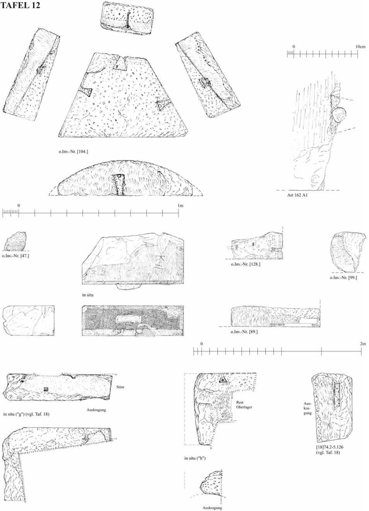
Säulenflickstück, Quader in situ , Quaderfragmente und fragmentarische Geisa – Kat. 8, 9, 119 a und 7 ohne Kat.-Nr. (3 × in situ , [18]74.2-5.126; ohne Inv.-Nr. [47.], [89.], [99.], [104.], [128.]; Art 162 A1) – [104.], [47.], [99.] im M. 1 : 10, die restlichen M. 1 : 20
