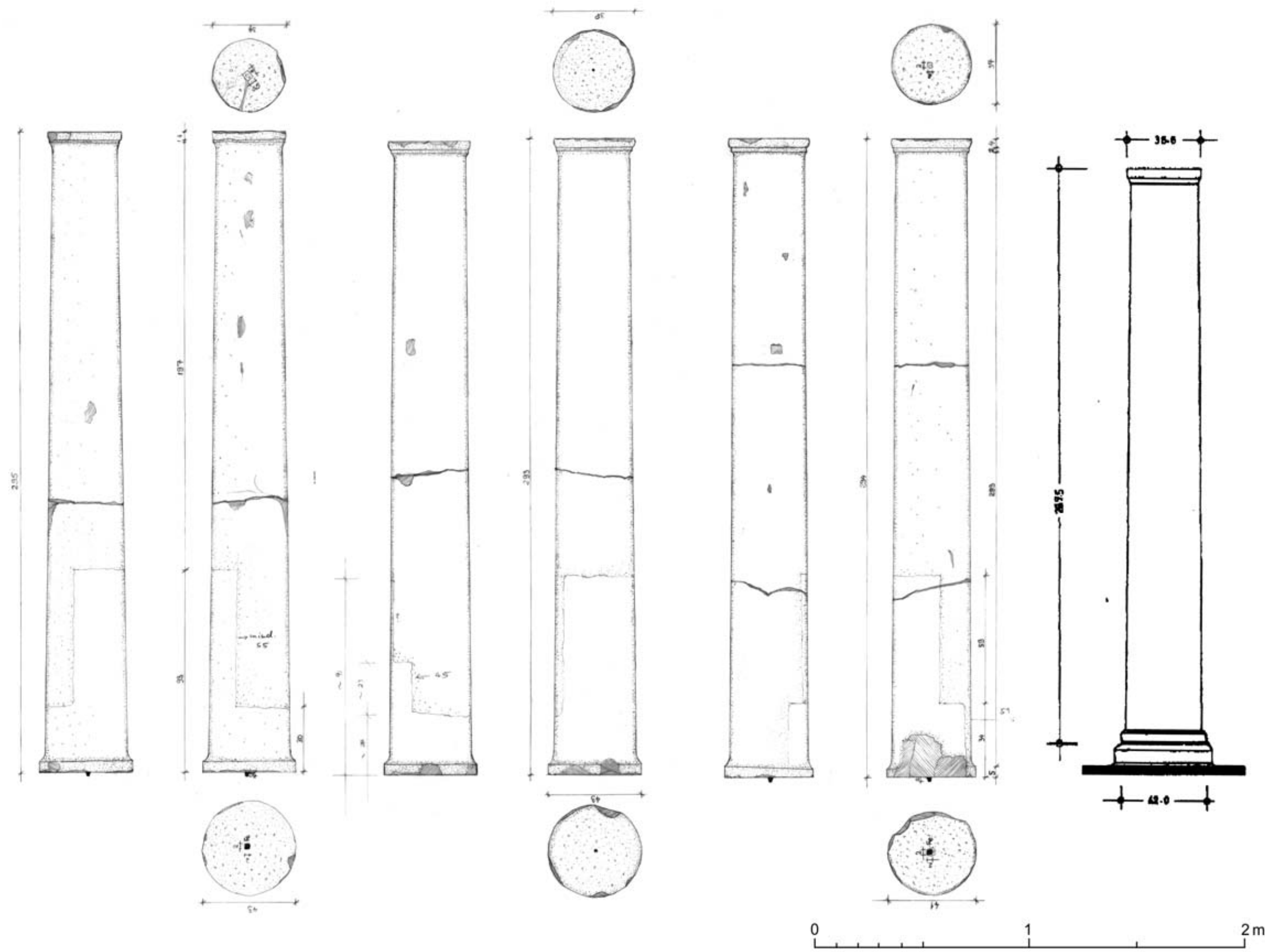
121.1: Säule A 17 (M 1:20)
