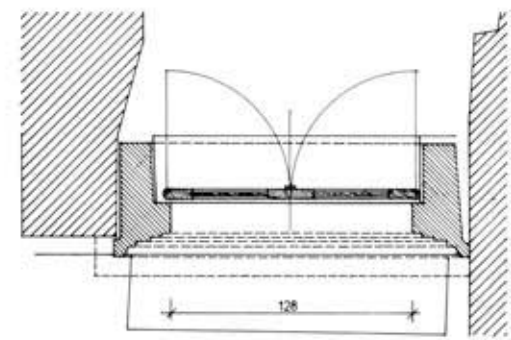
118.3: Rekonstruktion T 1 Eingangportal (M 1:40)
