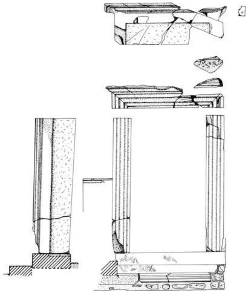
118.1: Marmorürgewände (M 1:40)
