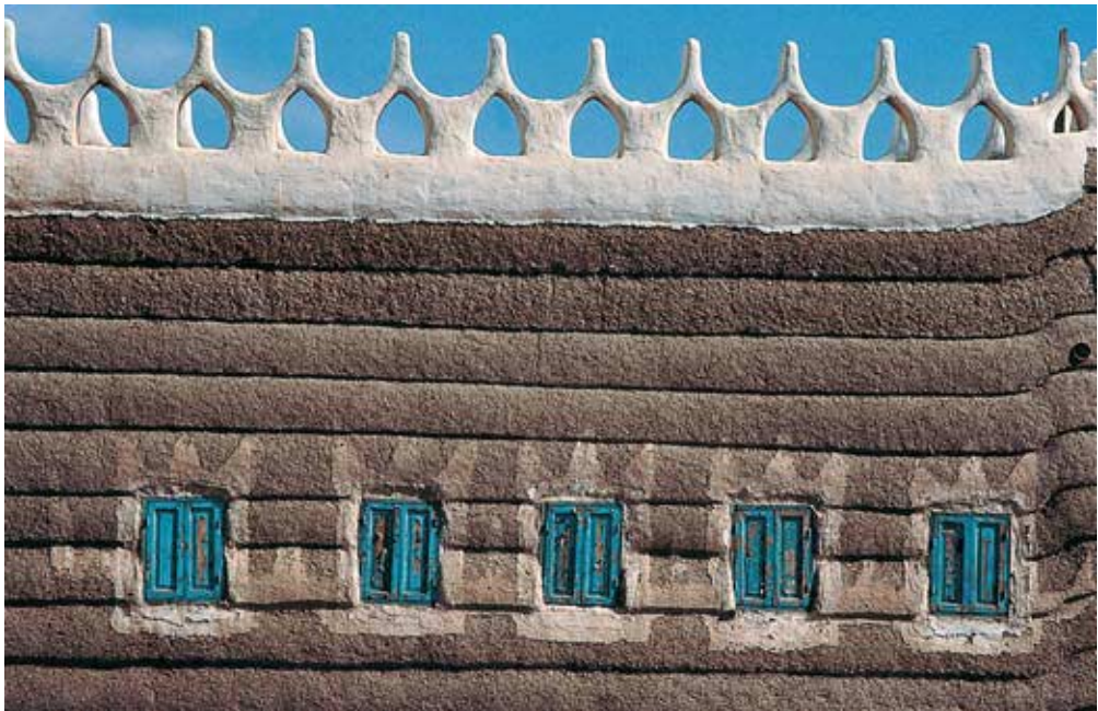
Abb. 87: Details einer Mauerkrone, W. Najrān
