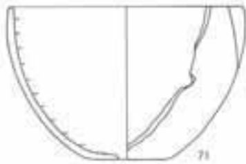
V 841 Tot. 105/3 M 1:4
