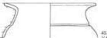
V 2784 Taf. 84/5, Nr. 16090 M 1:8
